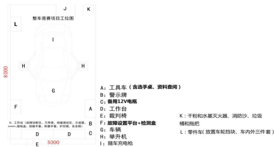
图 1 新能源汽车故障诊断与排除竞赛工位布置图
